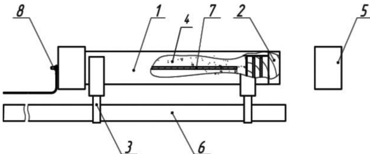
Рис.1 Медносульфатный неполяризующийся электрод сравнения переносной ЭНЕС-5М 1- корпус электролитической камеры, 2- пористый наконечник (дерево), 3- держатель рукоятки-удлинителя, 4- насыщенный раствор медного купороса, 5- заглушка пористого наконечника, 6- рукоятка-удлинитель, 7- контактный стержень из красной меди, 8- проводник – кабельный вывод.
